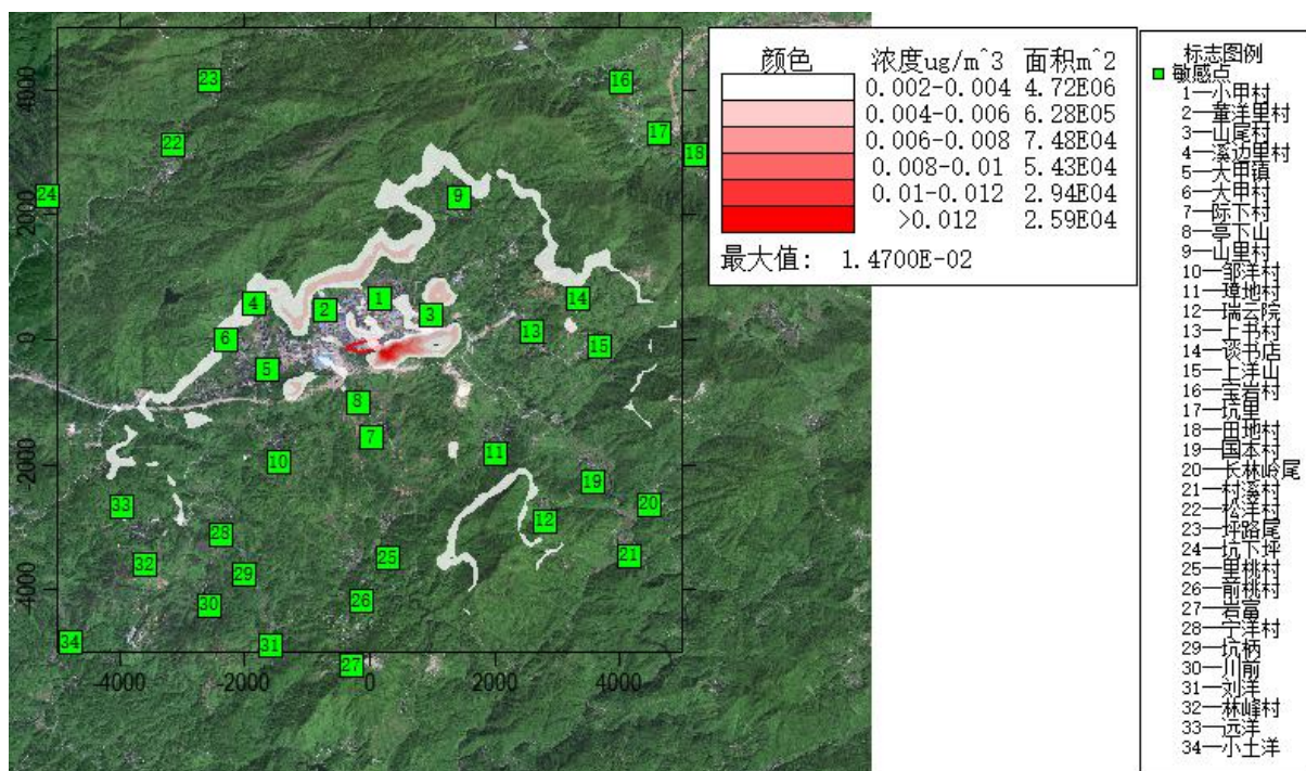
附图 6.1-28 锡叠加后小时浓度分布图
