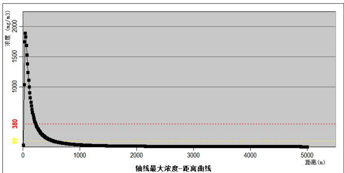
图 6.8-2 不利气象条件下 CO 轴线/质心最大浓度-距离曲线图 表 6.8-21 铝灰受潮氨气泄漏事故源项及事故后果基本信息表
