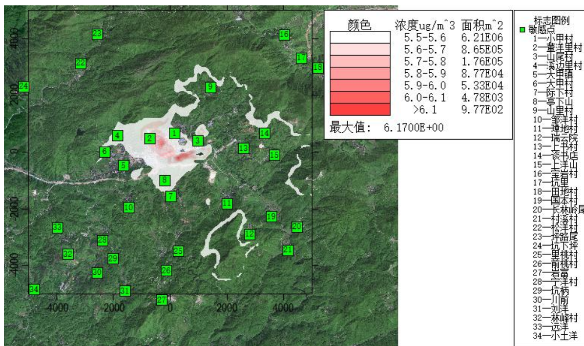
附图 6.1-8 \text{SO}_2 叠加后年均浓度分布图
