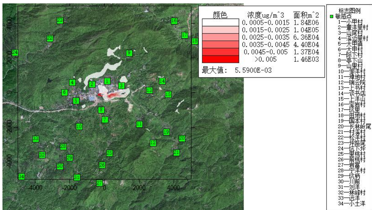
附图 6.1-17 HCl 日均浓度贡献值分布图
