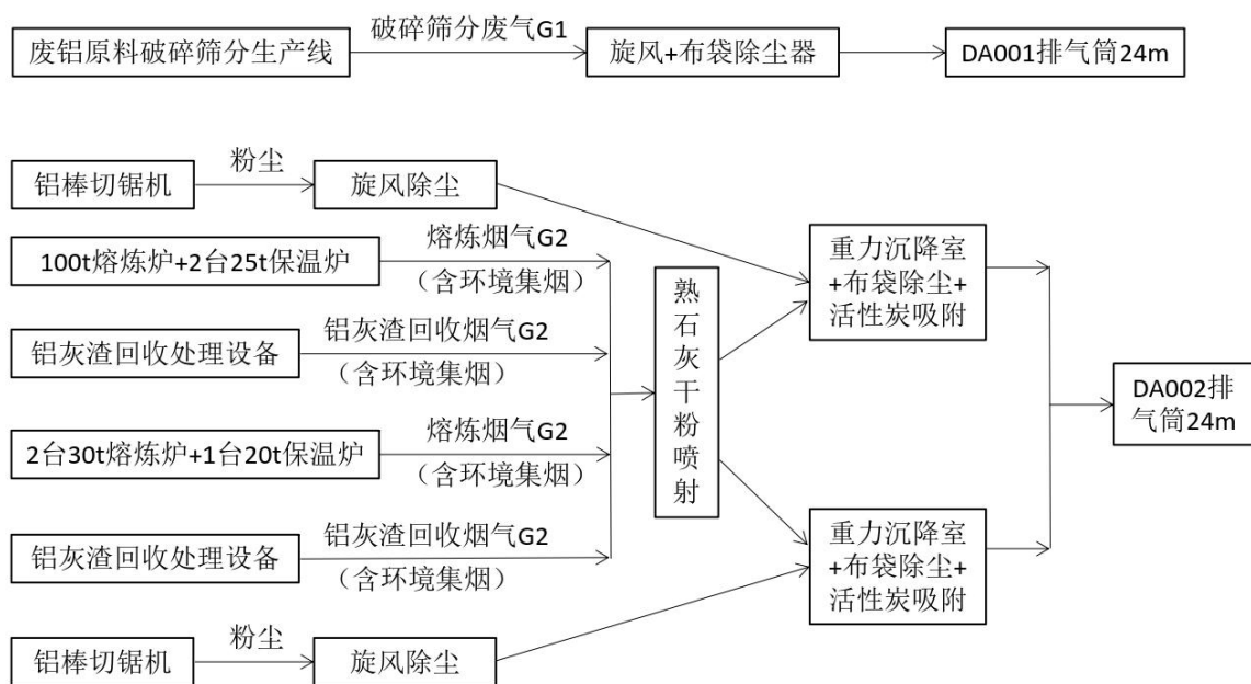
图 3.2-1 现有工程废气治理工艺流程图
