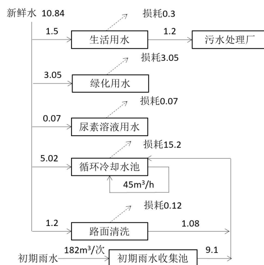
图 4.2-4 本项目水平衡图 单位 m 3 /d
