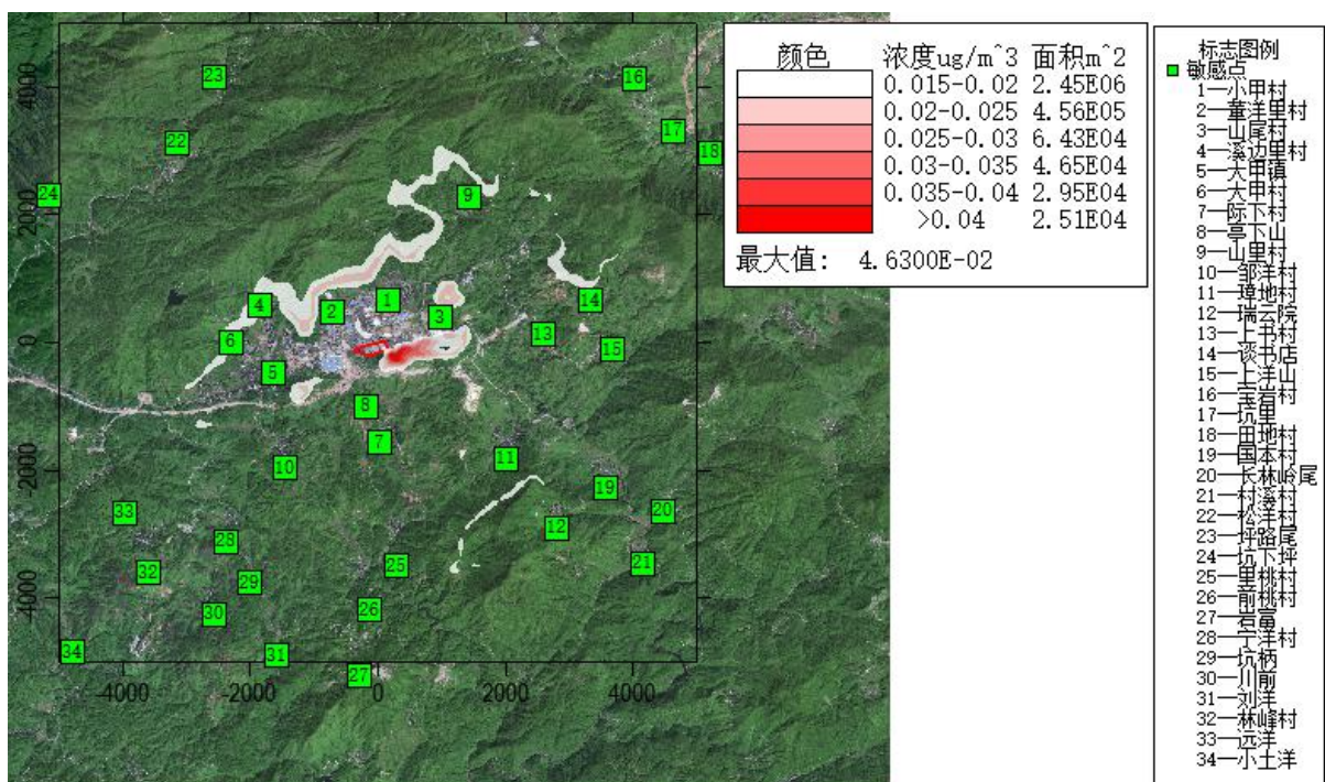
附图 6.1-16 HCl 叠加后小时浓度分布图
