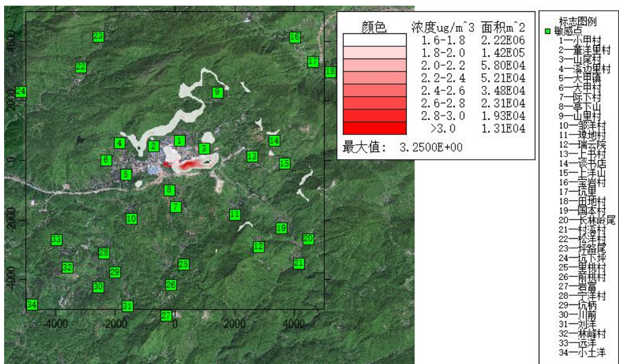
附图 6.1-19 氟化物叠加后日均浓度分布图
