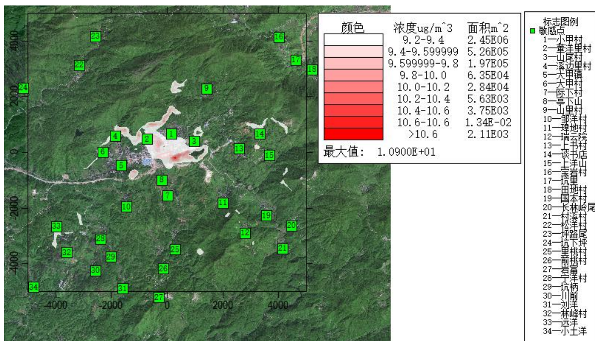
附图 6.1-7 \text{SO}_2 叠加后 98%保证率日均浓度分布图
