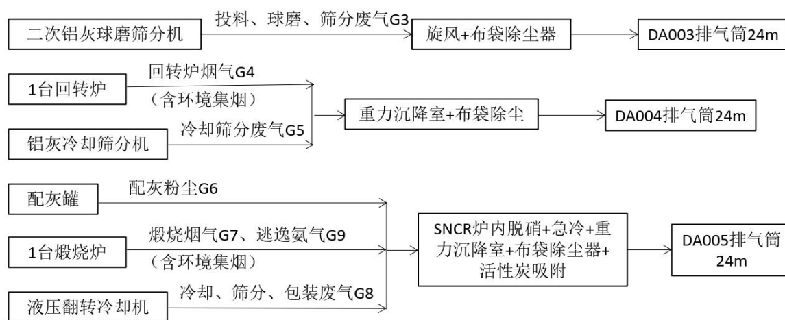
图 7.2-1 主要废气治理工艺流程图
