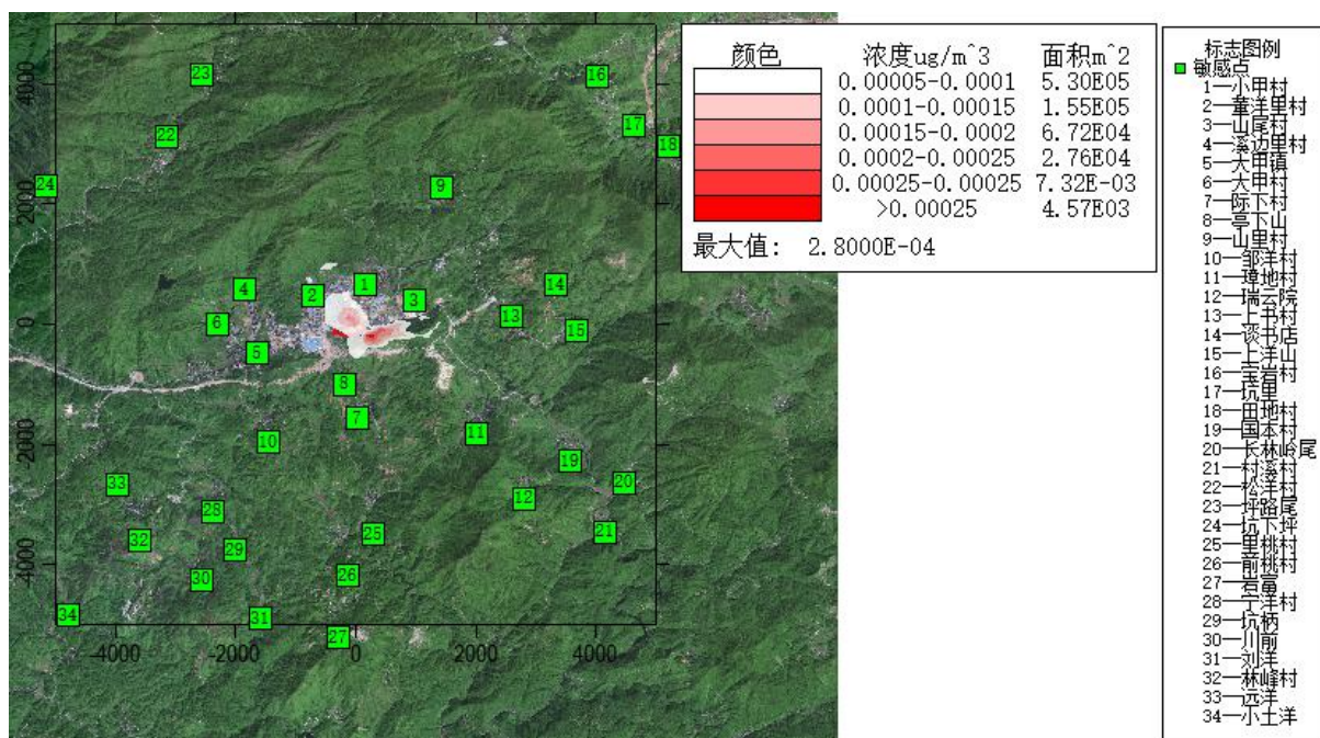
附图 6.1-25 砷年均浓度贡献值分布图
