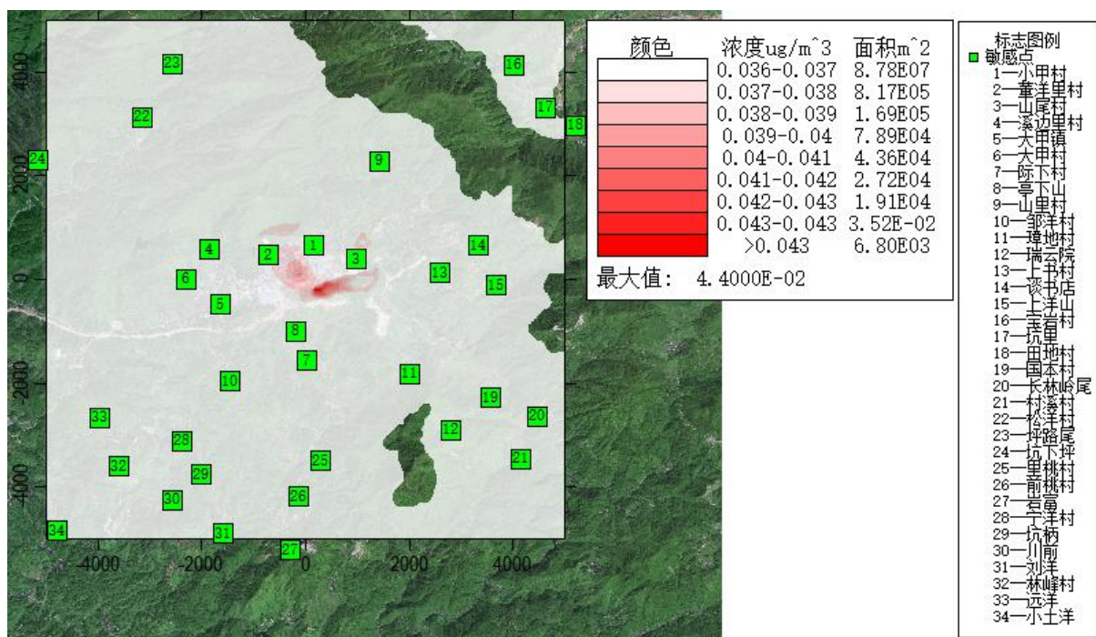
附图 6.1-31 二噁英年均浓度贡献值分布图
