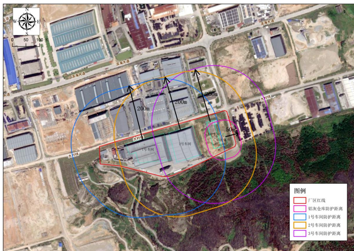
图 6.1-32 项目建成后全厂环境防护距离包络图
