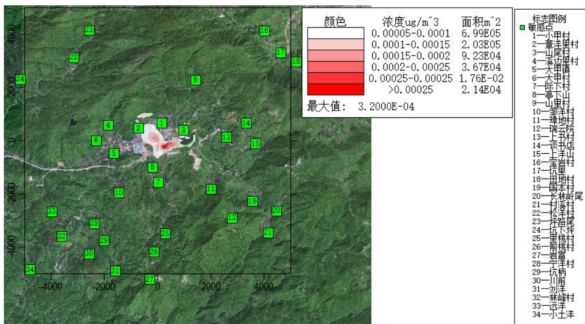
附图 6.1-21 铅年均浓度贡献值分布图
