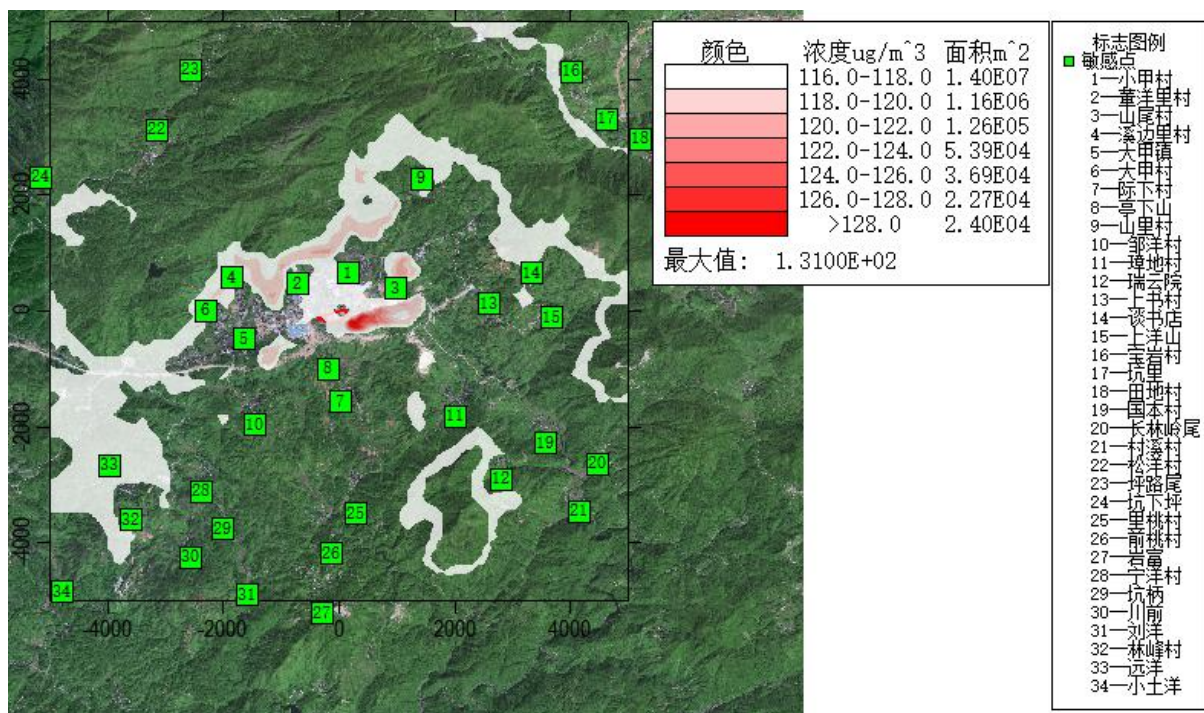
附图 6.1-32 氨叠加后小时浓度分布图
