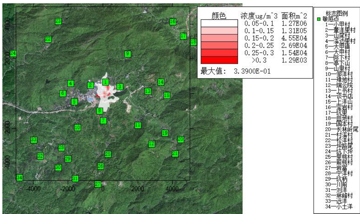
附图 6.1-29 锰及其化合物叠加后日均浓度分布图
