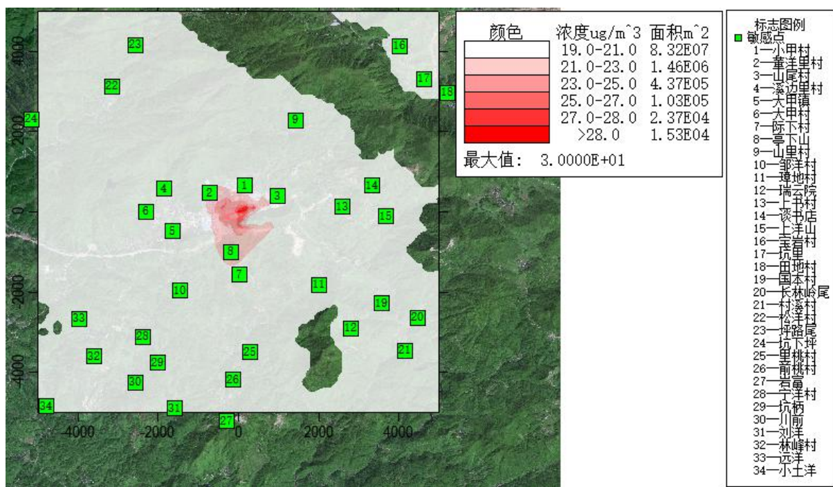
附图 6.1-14 \text{PM}_{2.5} 叠加后年均浓度分布图
