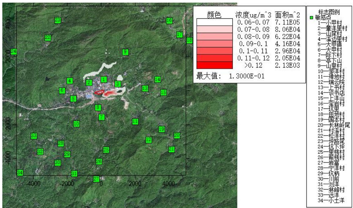
附图 6.1-30 二噁英叠加后日均浓度分布图
