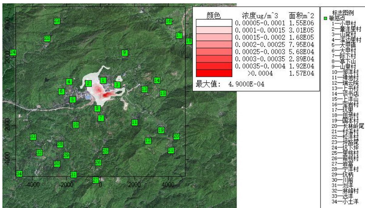
附图 6.1-27 汞年均浓度贡献值分布图
