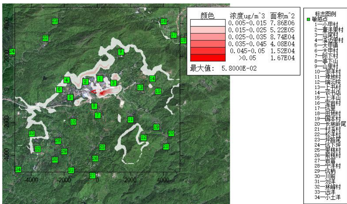
附图 6.1-22 铅叠加后小时浓度分布图
