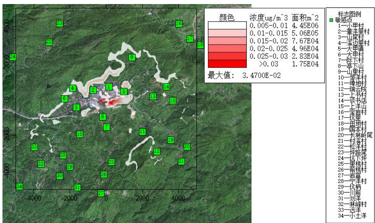
附图 6.1-26 汞叠加后小时浓度分布图
