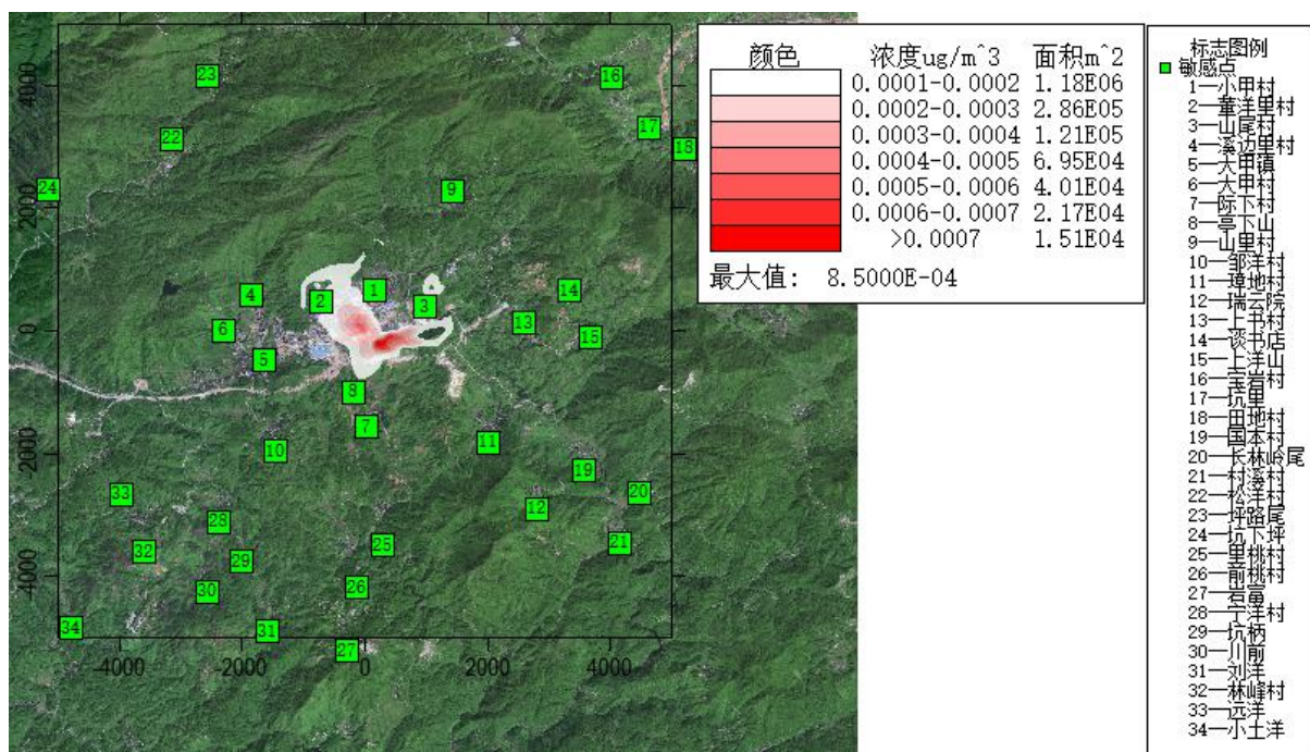
附图 6.1-23 铅年均浓度贡献值分布图
