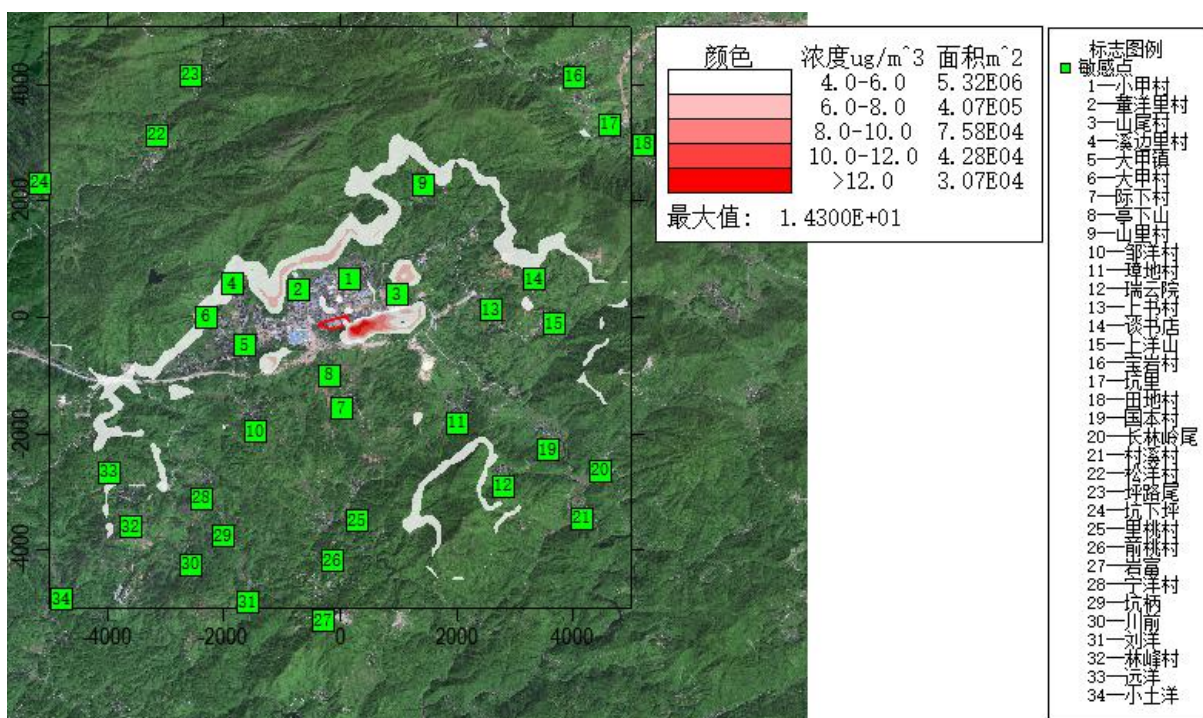
附图 6.1-18 氟化物叠加后小时浓度分布图
