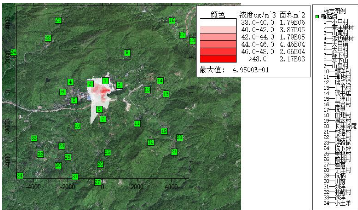
附图 6.1-13 \text{PM}_{2.5} 叠加后 95%保证率日均浓度分布图
