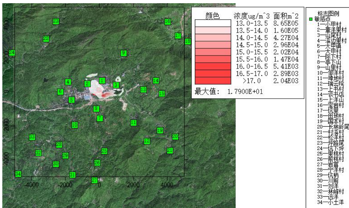
附图 6.1-10 \text{NO}_2 叠加后年均浓度分布图
