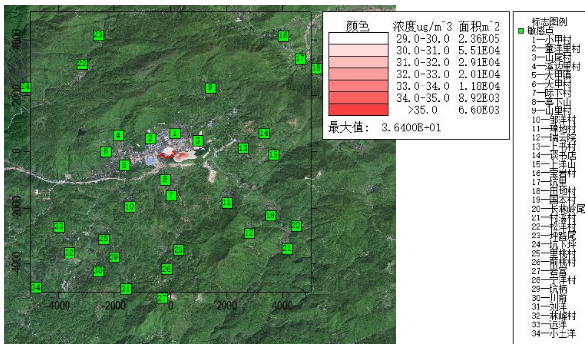
附图 6.1-9 \text{NO}_2 叠加后 98%保证率日均浓度分布图
