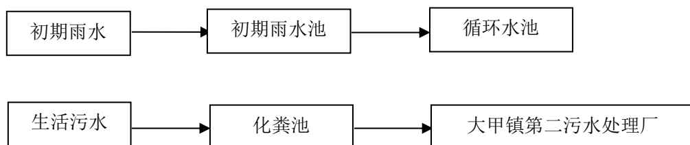
图 3.2-4 现有工程废水治理工艺流程图
