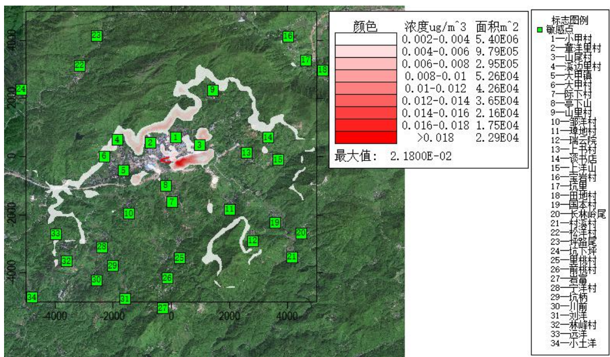
附图 6.1-20 镉叠加后小时浓度分布图
