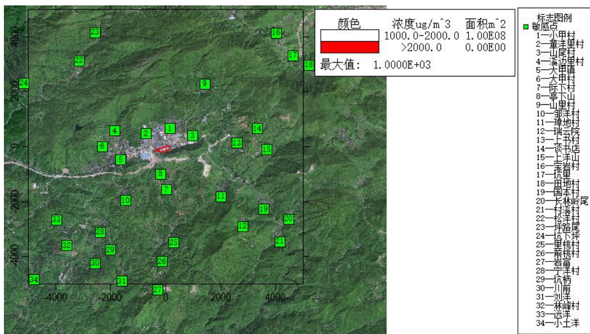
附图 6.1-15 CO 叠加后年均浓度分布图
